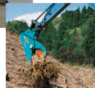
ウッドシヤ 樹木の伐採・抜根・切断・積込、木造家屋・船の解体、ロール紙の切断等さまざまな作業に威力を発揮します。
